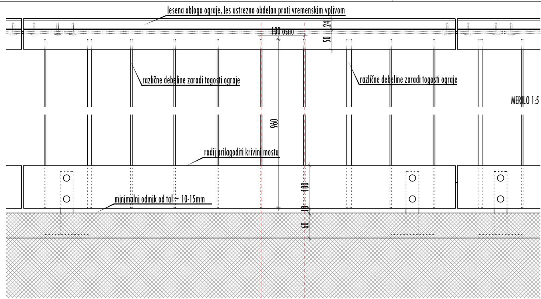
MERILO 1:5
