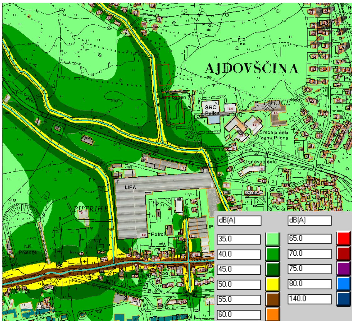
Slika 8: dnevni hrup lokalnih prometnic
