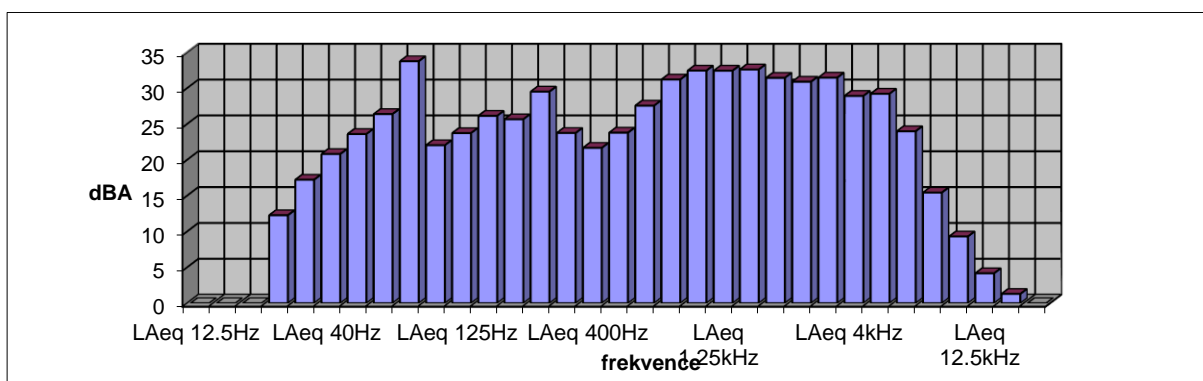
Slika 6: tipični frekvenčni spekter
