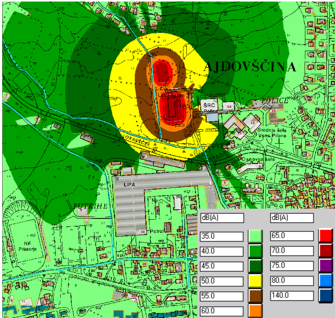
Slika 9: dnevni hrup športnih površin
