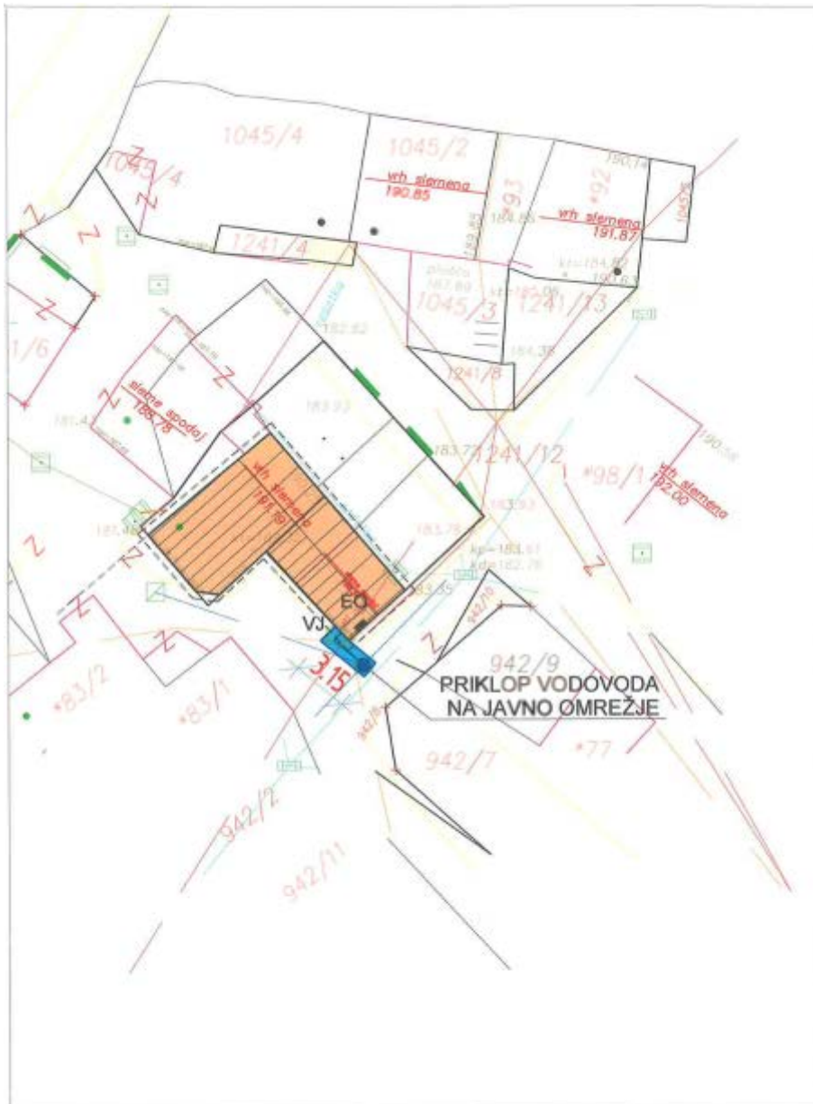
SKICA POTEKA VODOVODA PARCELA 1241/12 k.o. SKRILJE MERILO 1:250
