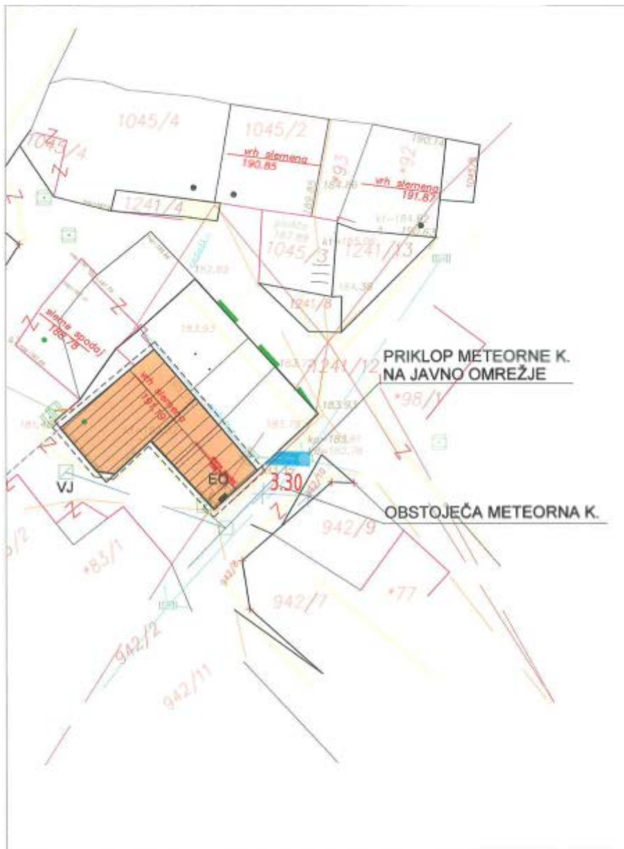
SKICA POTEKA METEORNE KANALIZACIJE PARCELA 1241/12 k.o. SKRILJE MERILO 1:250
