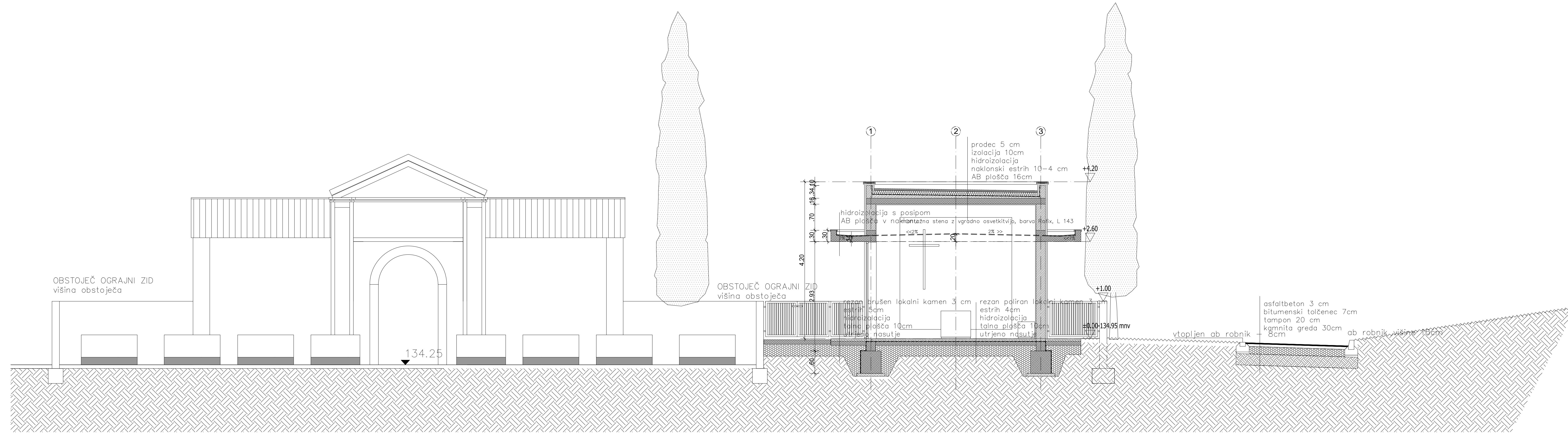
PREREZ AA
