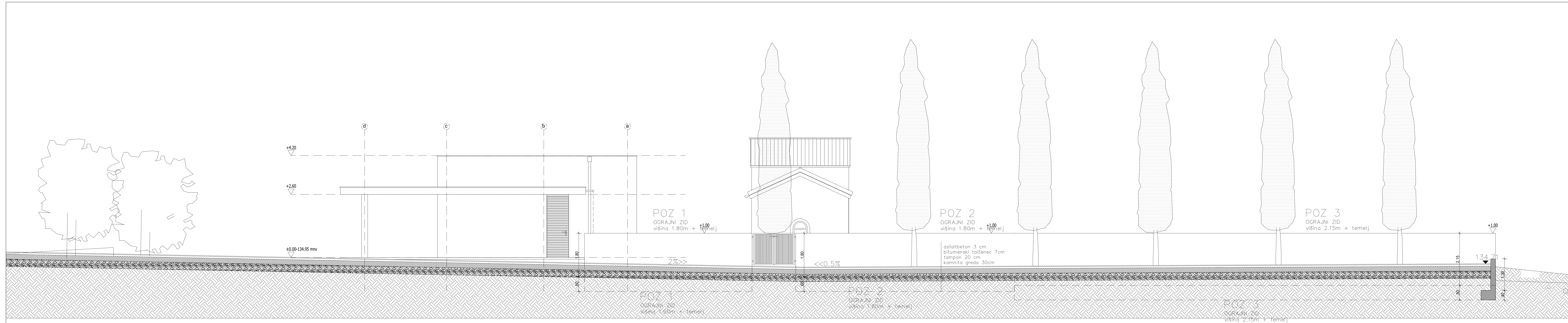
SEVEROVZHODNA FASADA – POGLED IZ DOVOZNE CESTE IN PARKIRIŠČA
